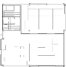
25 Bauplan Umbrella House © DEHLI GROLMUND. Alle Umbrella House Pläne wurden auf Grundlage der originalen Werkpläne angefertigt und mit dem Kazuo Shinohara Estate abgestimmt.
