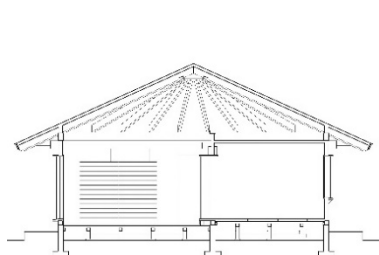
22 Bauplan Umbrella House © DEHLI GROLMUND Alle Umbrella House Pläne wurden auf Grundlage der originalen Werkpläne angefertigt und mit dem Kazuo Shinohara Estate abgestimmt.
